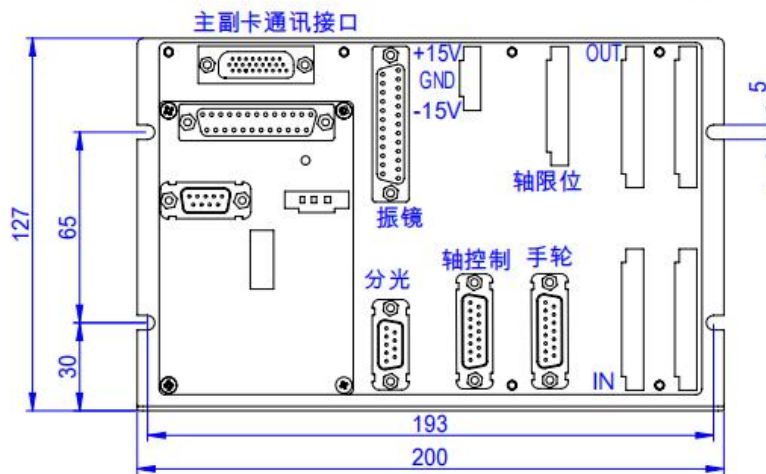
PCIE 端子板
