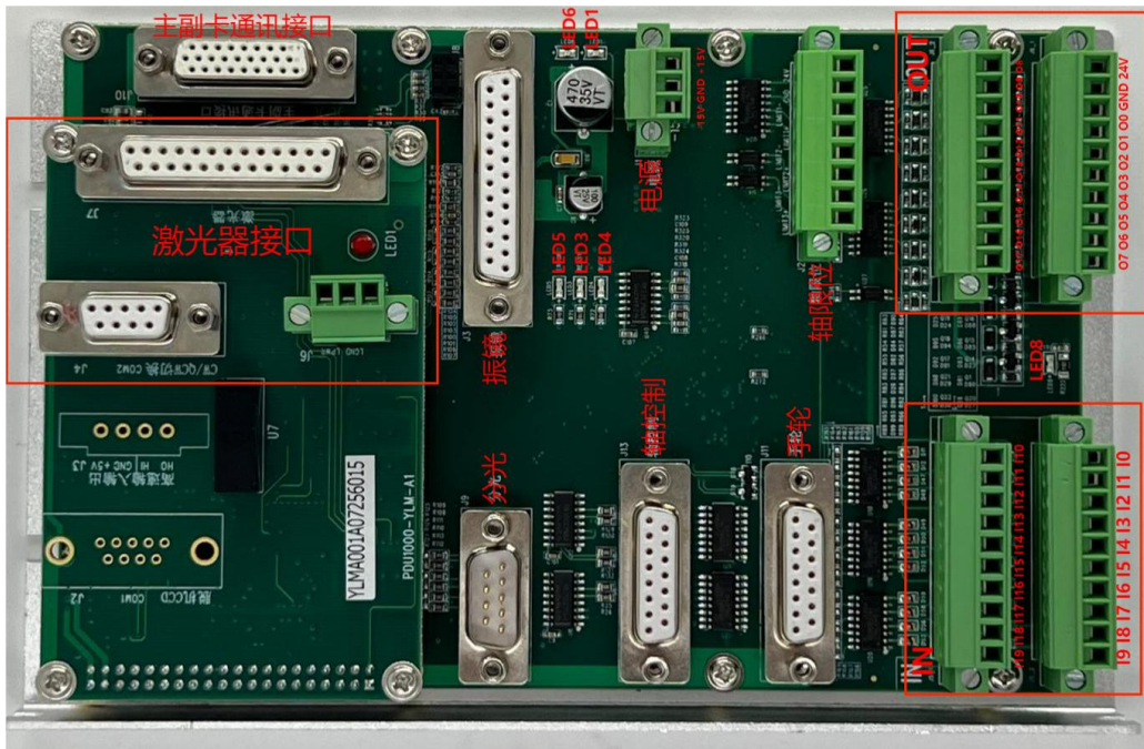
PCIE 端子板
