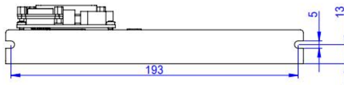
PCIE 主卡
